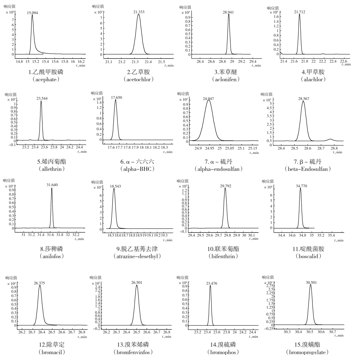
图 C.1 A、B 两组农药和内标物多反应监测(MRM)色谱图
